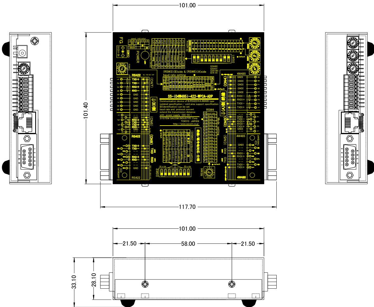
本体寸法図
