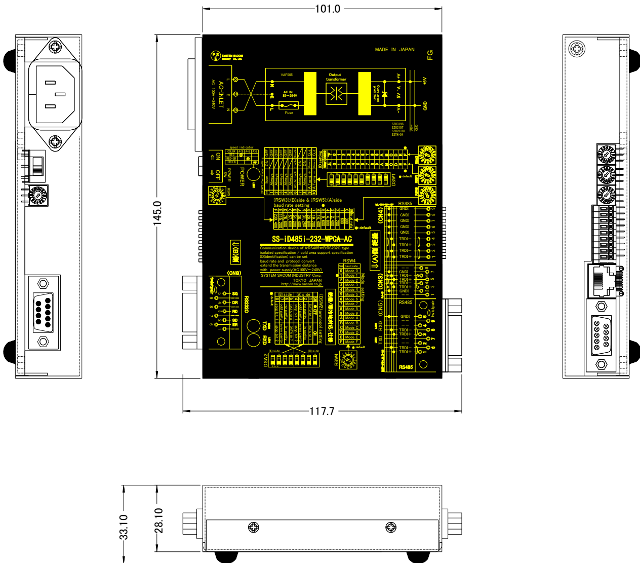
本体寸法図
