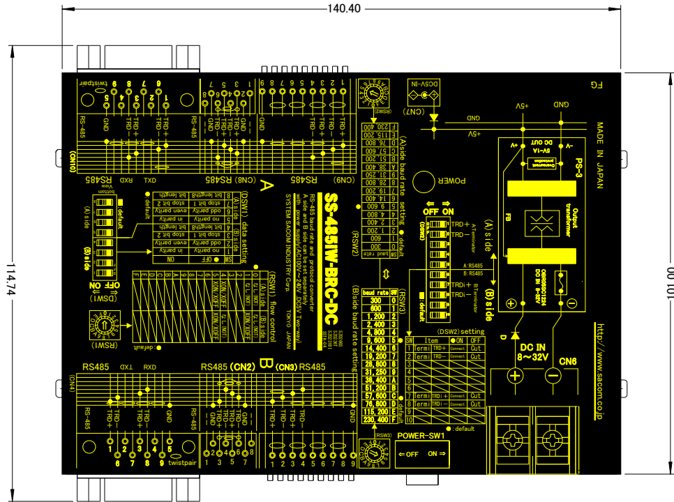
本体寸法図
