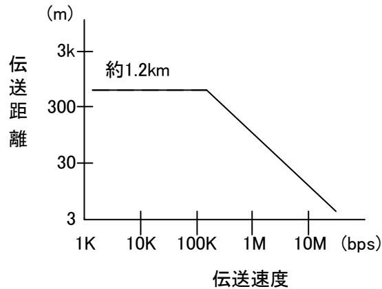
参考図 RS485 と RS485 の伝送速度と伝送距離の関係(グラフは両対数目盛り)
