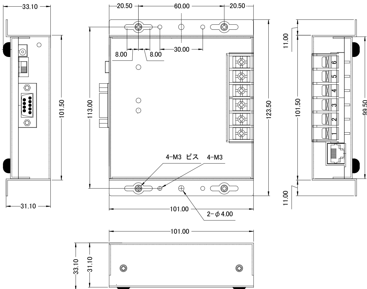
寸法図
