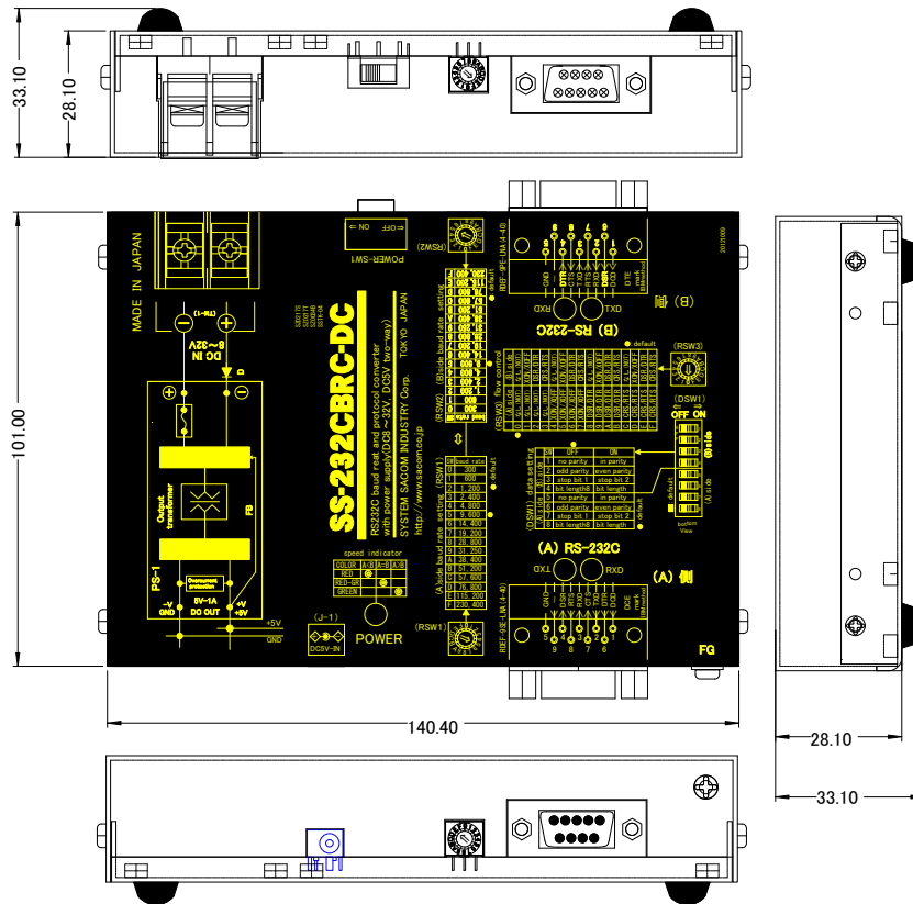
本体寸法図
