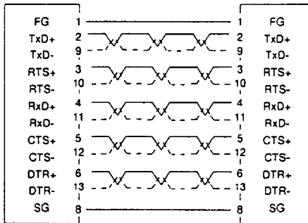
1対1接続ケーブル結線(ストレートケーブル)
