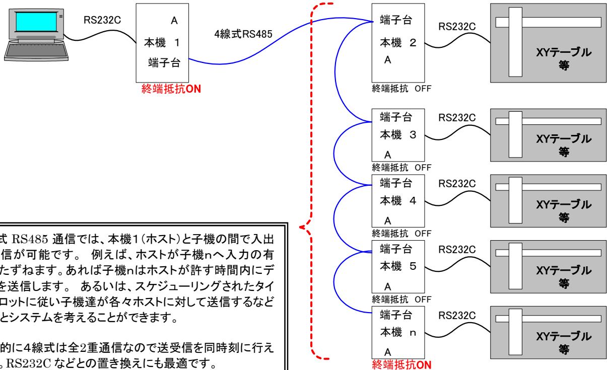
1:n接続例
